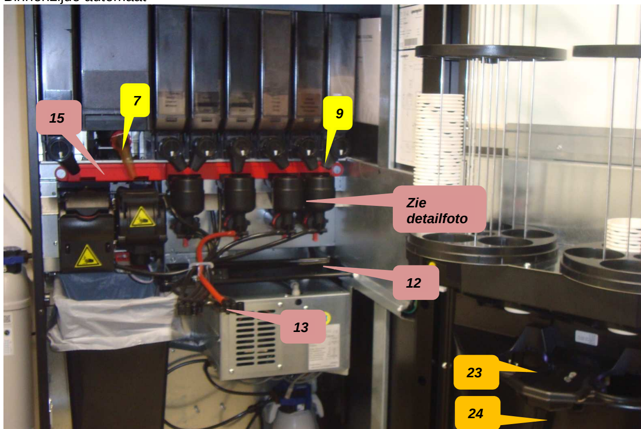
Binnenzijde automaat
