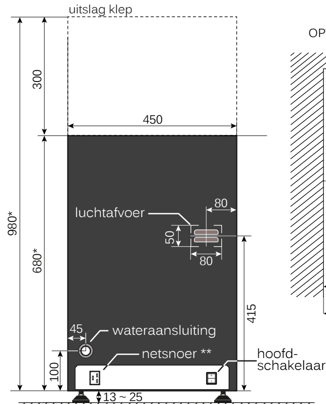
[ACHTERAANZICHT AUTOMAAT]
