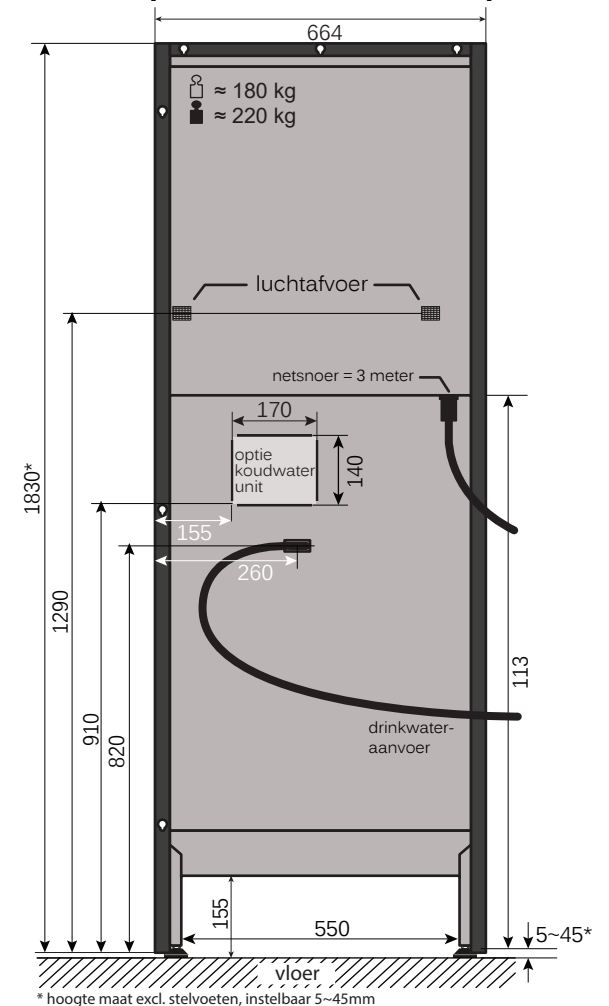
[ ACHTERAANZICHT AUTOMAAT ]
