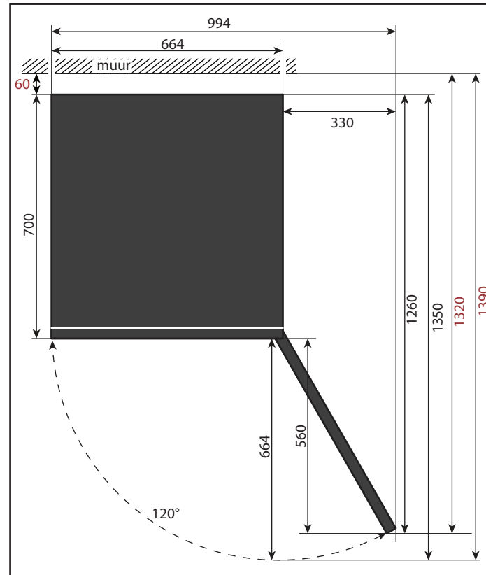
[ BOVENAANZICHT AUTOMAAT ]
